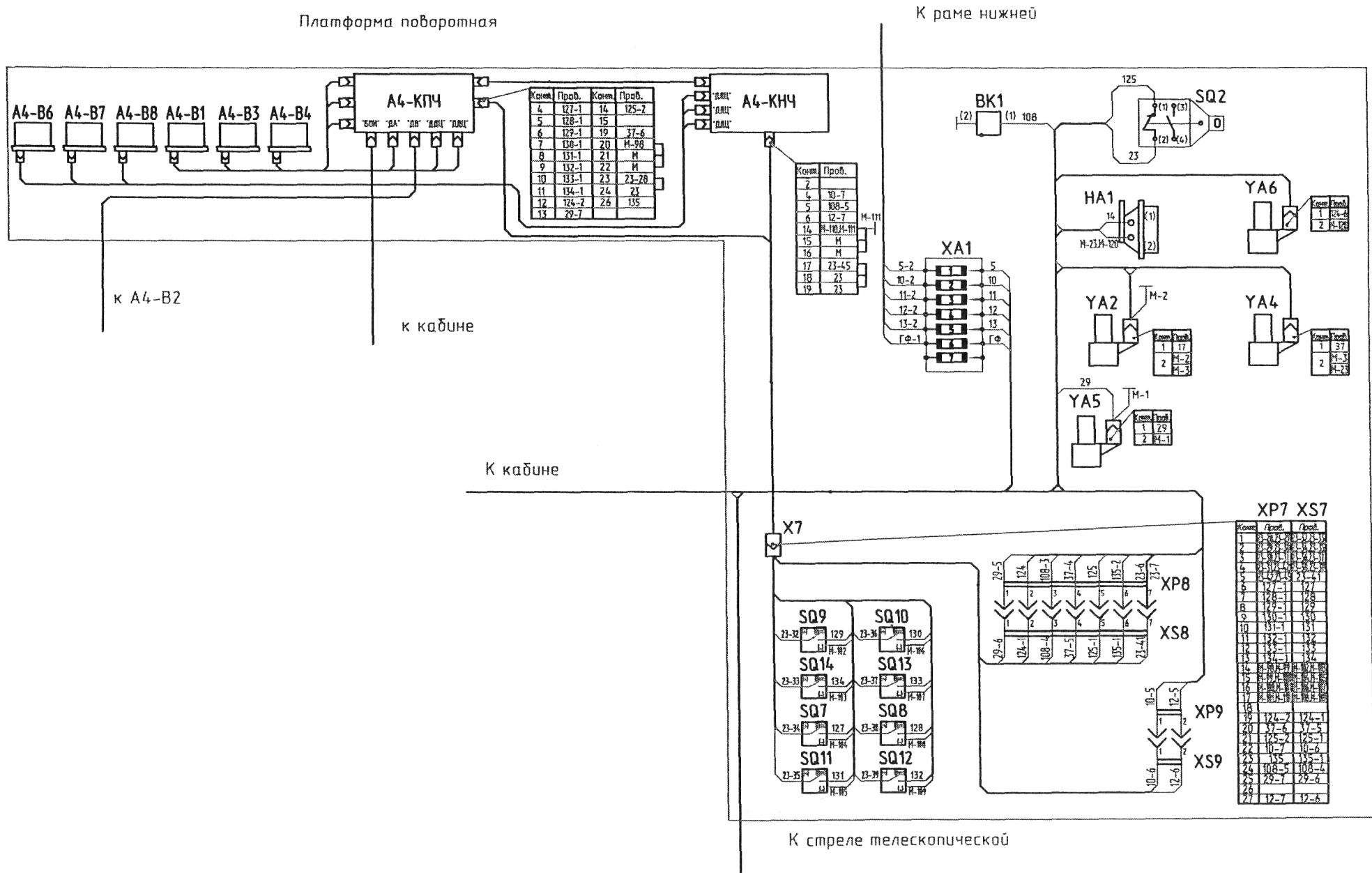
Рисунок 44-Схема электрическая соединений крана KC-55727-1 (лист 4)
