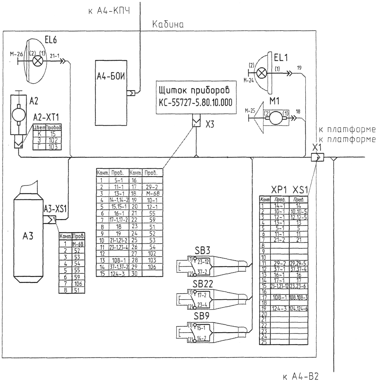
Рисунок 44-Схема электрическая соединений крана КС-55727-1 (лист 3)
