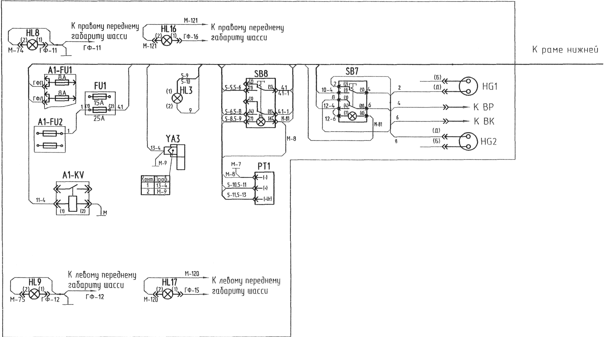
Рисунок 44 - Схема электрическая соединений крана КС-55727-1 (лист 1)
