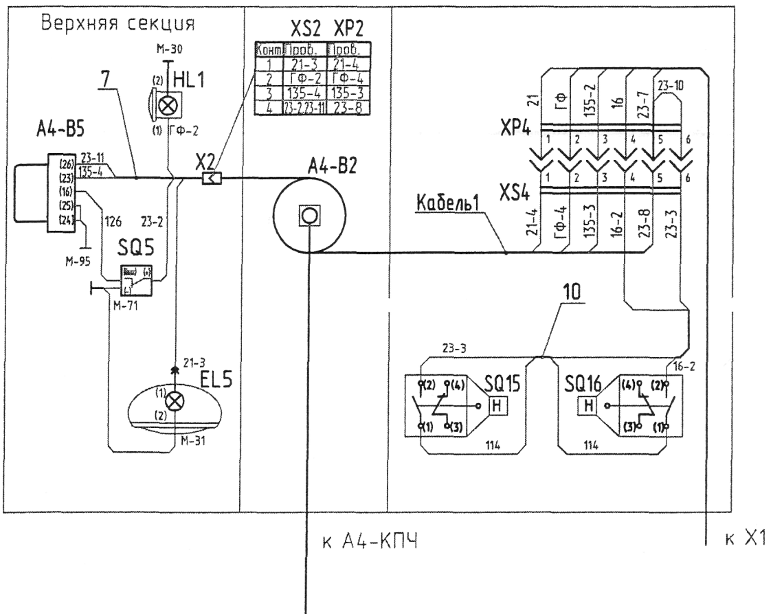
Рисунок 44- Схема электрическая соединений крана КС-55727-1 (лист 2)
