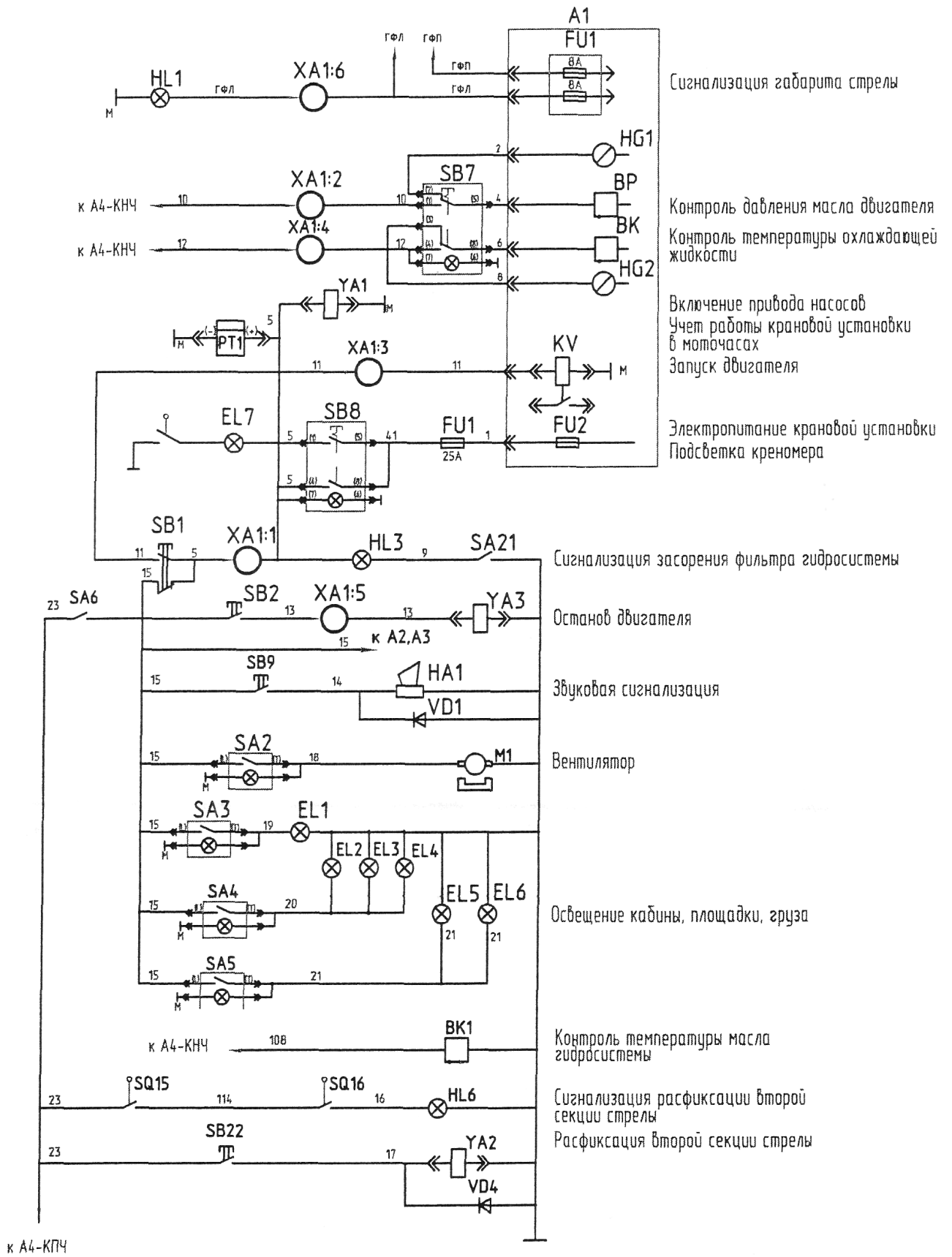
Рисунок 43 - Схема электрическая принципиальная автокрана КС-55727-1 (лист 1)
