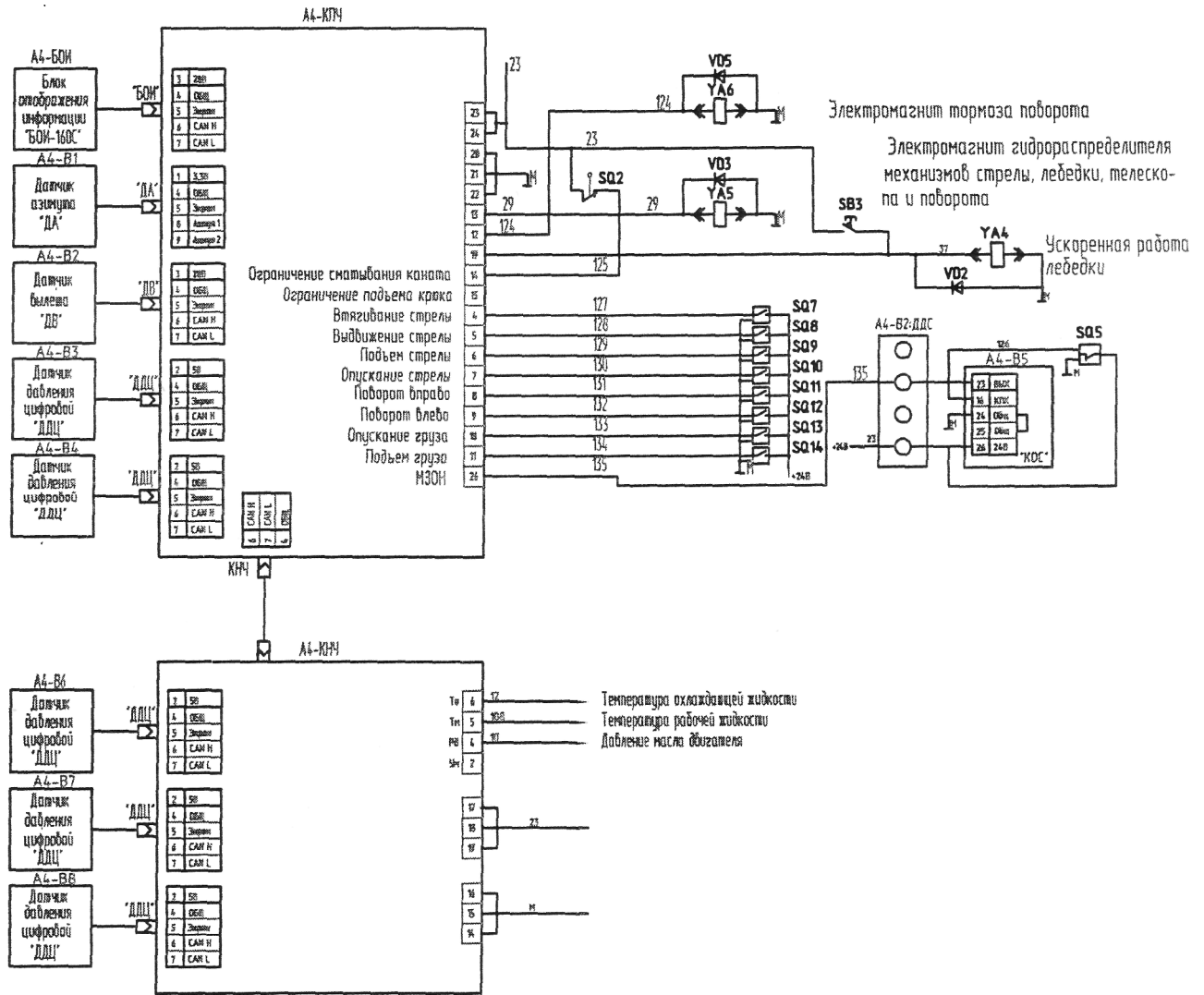
Рисунок 43 - Схема электрическая принципиальная автокрана КС-55727-1 (лист 2)
