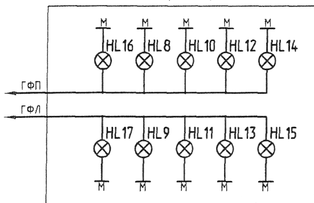
Рисунок 43 - Схема электрическая принципиальная автокрана КС-55727-1 (лист 3)
